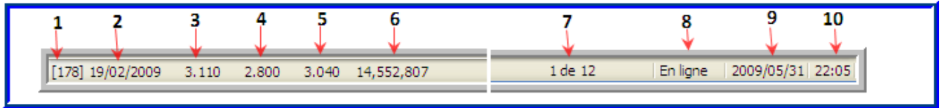
Figure 6.17 Barre d'état
