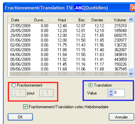
Figure 6.8 Fractionnement/Translation
